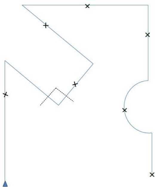
Obr.č.6 – Příklad tvarů stop IFH-2 (IGP-FH)
